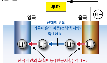
배터리 모식도
