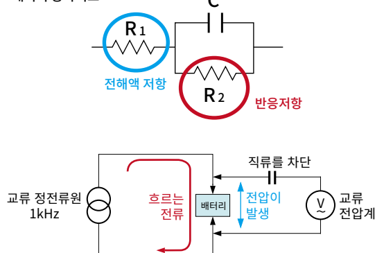
배터리 등가회로
