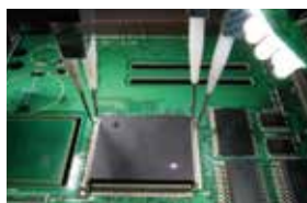
플라잉 프로브 테스터 FA1240 시리즈
