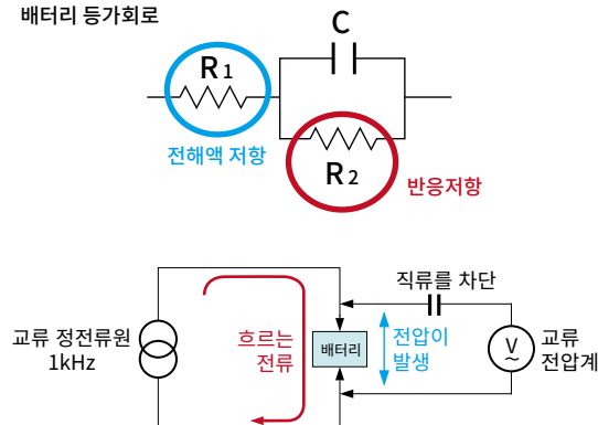
배터리 등가회로
