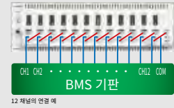
배터리 셀 전압 제너레이터 SS7081
